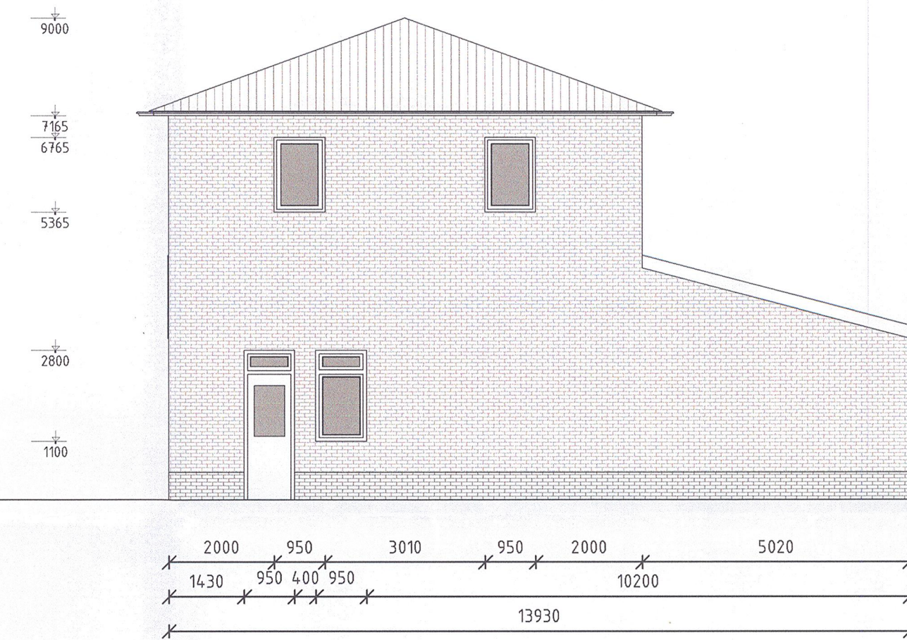
ZIJGEVEL (NOORD-OOST) SCHAAL 1:100
