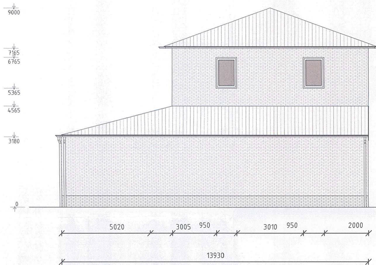
ZIJGEVEL (ZUID-WEST) SCHAAL 1:100
