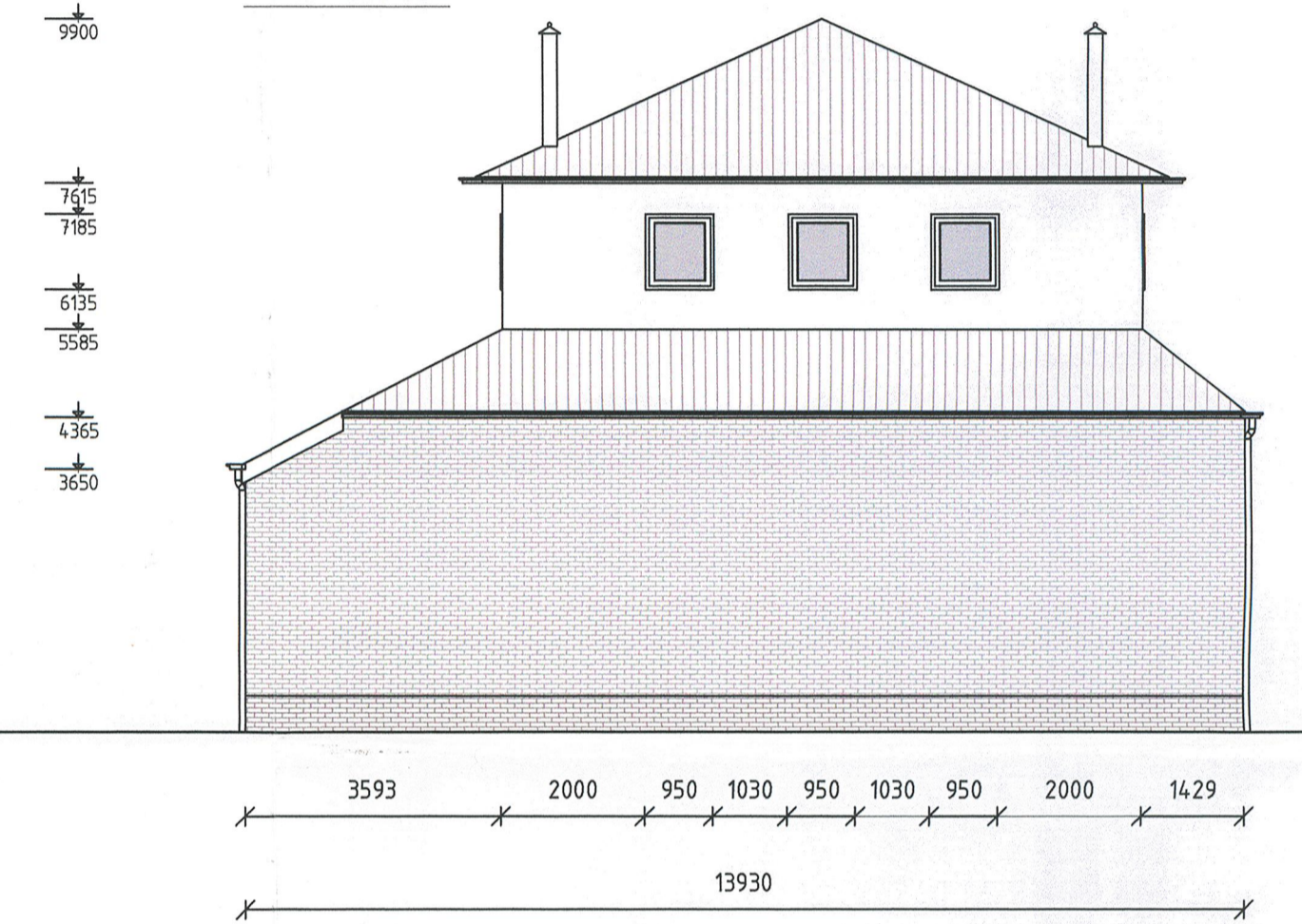
ACHTERGEVEL (NOORD-WEST) SCHAAL 1:100
