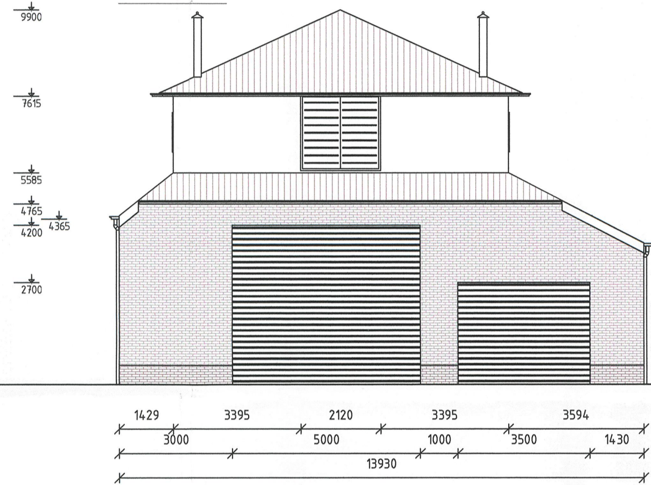
VOORGEVEL (ZUID-OOST) SCHAAL 1:100
