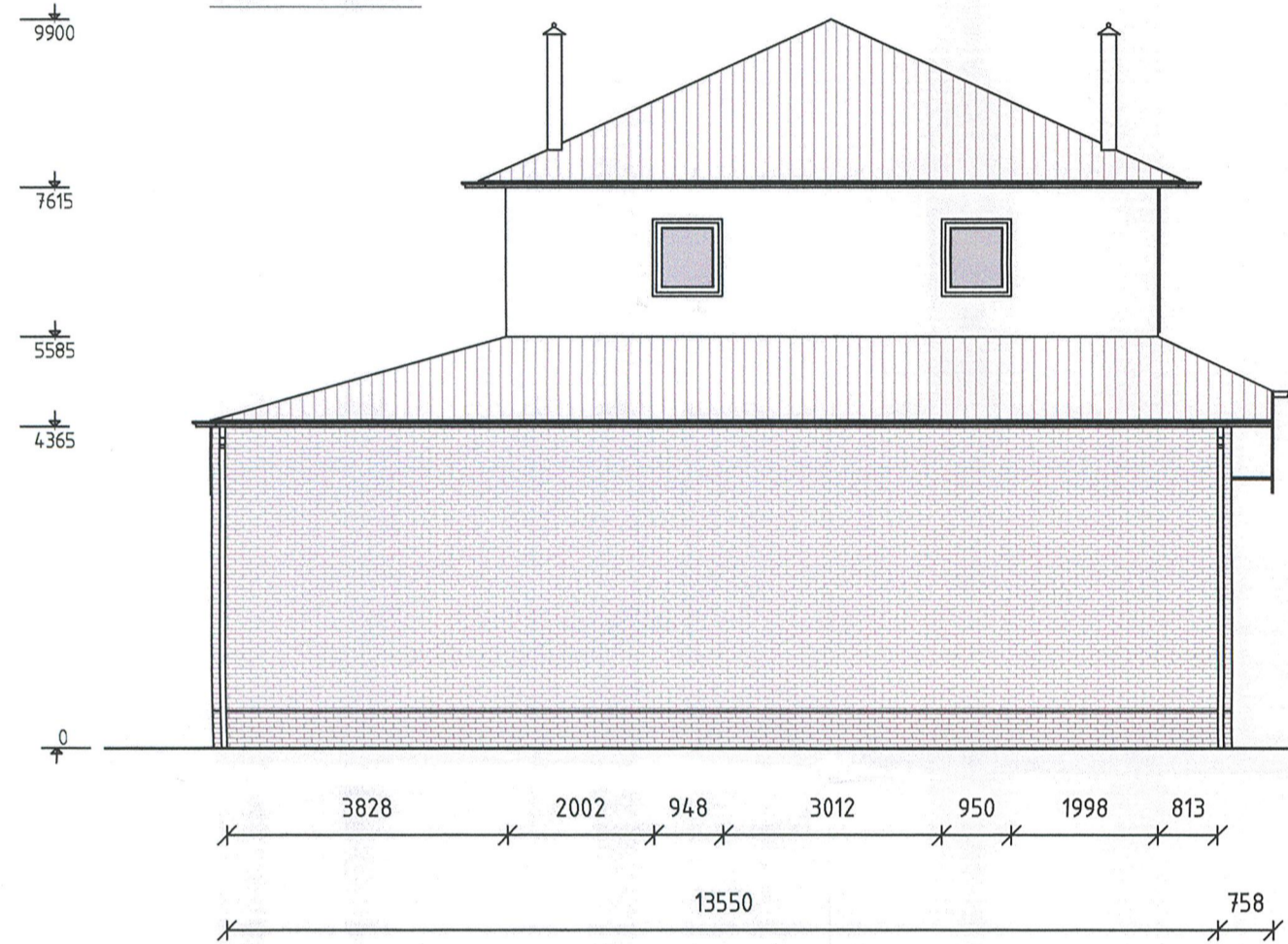
ZIJGEVEL (ZUID-WEST) SCHAAL 1:100
