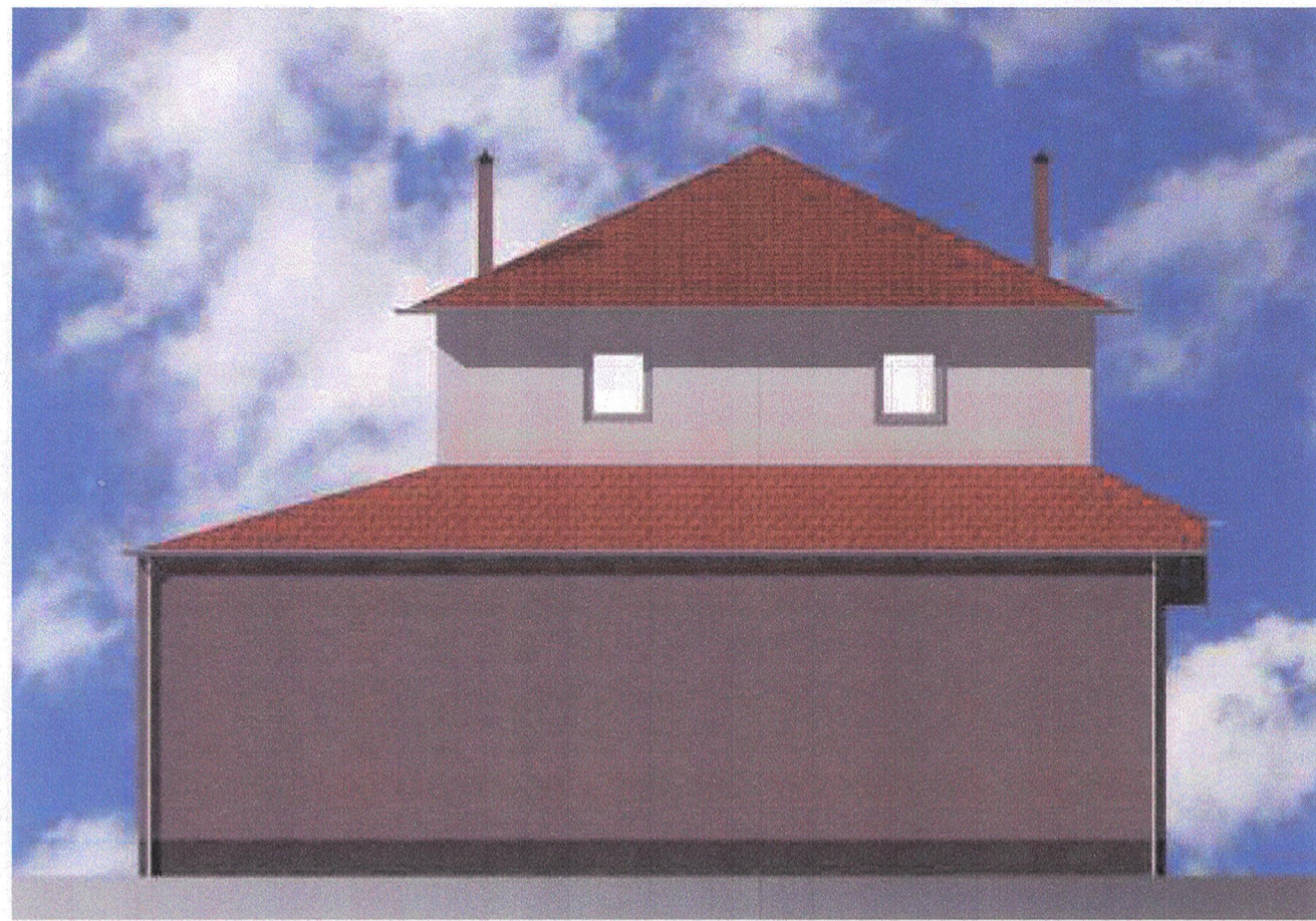
ZIJGEVEL (ZUID-WEST) SCHAAL 1:100
