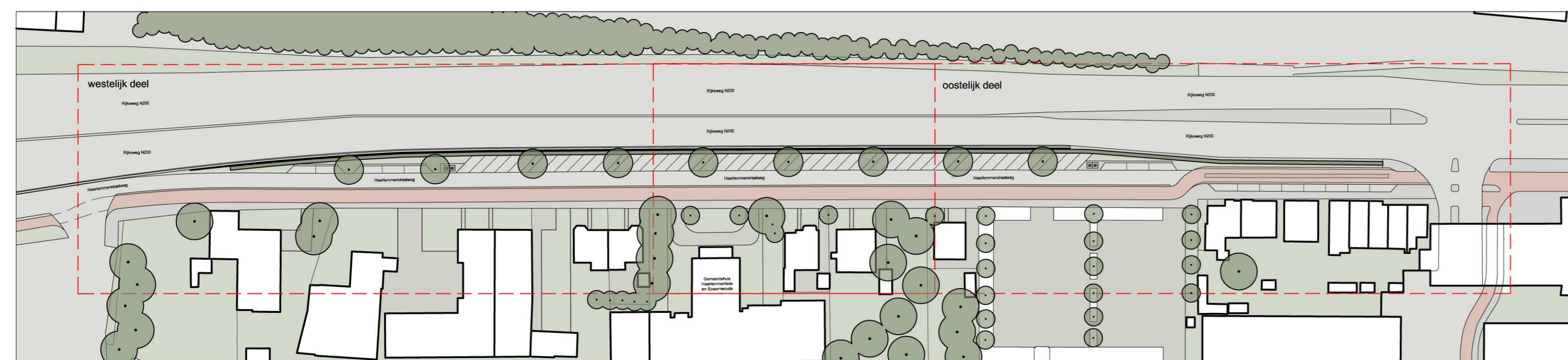
Overzichtstekening 1:1000
