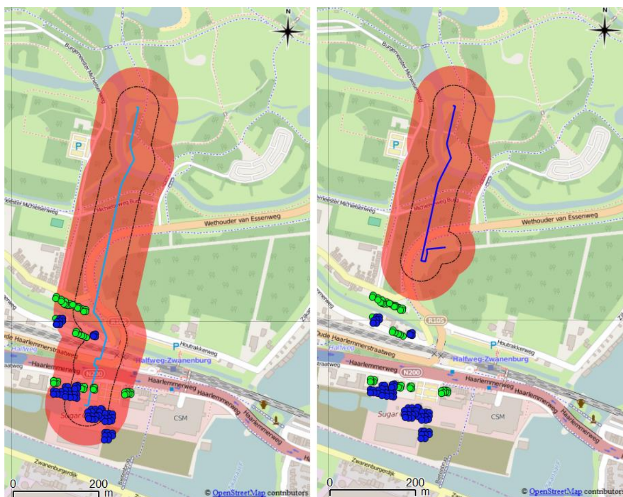
Figuur 2 Bevolkingsgegevens rondom de W-534-03 zoals aangeleverd door de populatieservice van IPO. Groen gekleurde punten zijn woningen, blauw gekleurde punten zijn werklocaties. Het rode gebied geeft het invloedsgebied (1% letaliteitsgrens) van de leiding weer; de stippellijn geeft de 100% letaliteitsgrens weer. Links wordt de huidige situatie weergegeven en rechts de toekomstige situatie.
