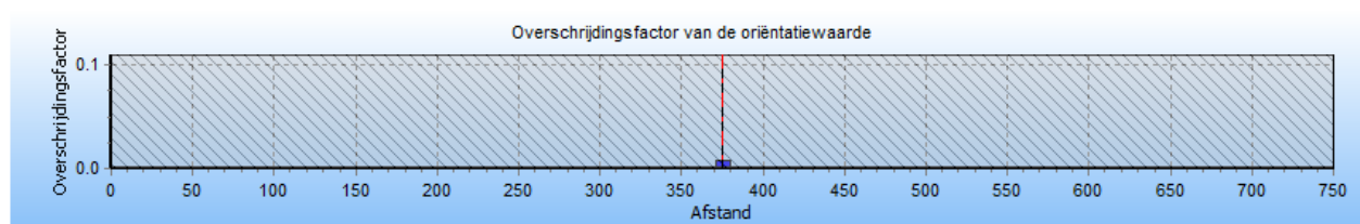
Figuur 5 Overschrijding van het groepsrisico als functie van de stationing van de W-534-03.
