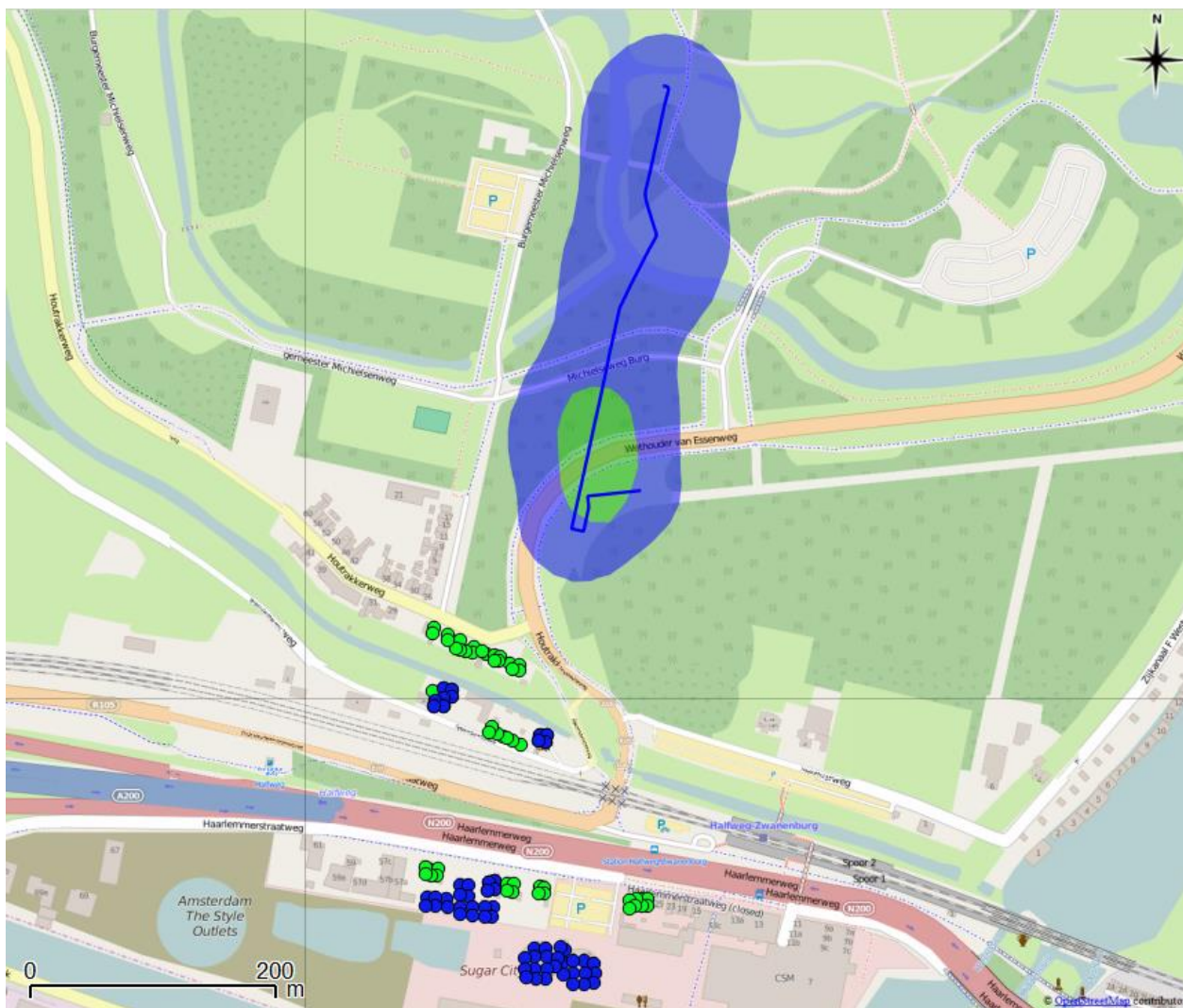
Figuur 4 Ligging van gastransportleiding W-534-03 (donkerblauw) in de toekomstige situatie. De plaatsgebonden risicocontouren rondom de leiding zijn, wanneer aanwezig, weergegeven met de volgende kleuren:
