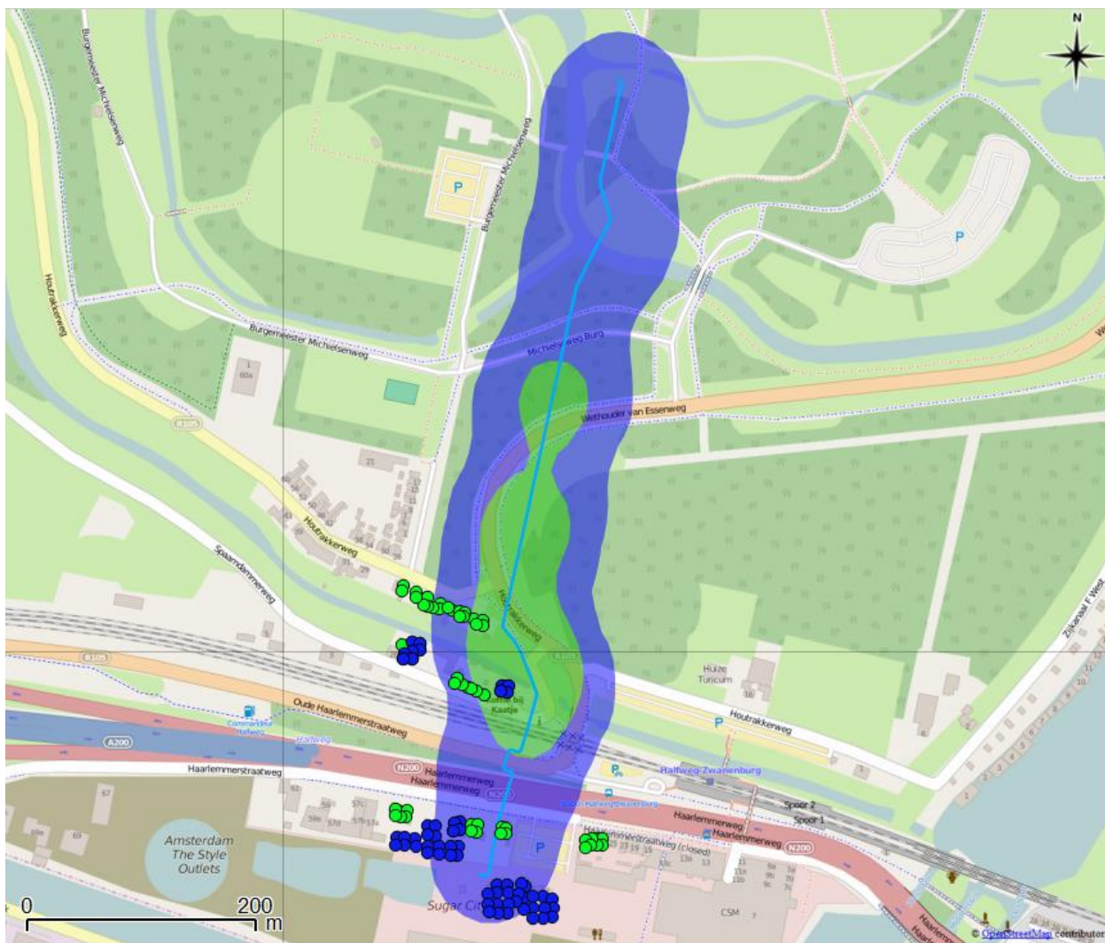
Figuur 3 Ligging van gastransportleiding W-534-03 (lichtblauw) in de huidige situatie. De plaatsgebonden risicocontouren rondom de leiding zijn, wanneer aanwezig, weergegeven met de volgende kleuren:
