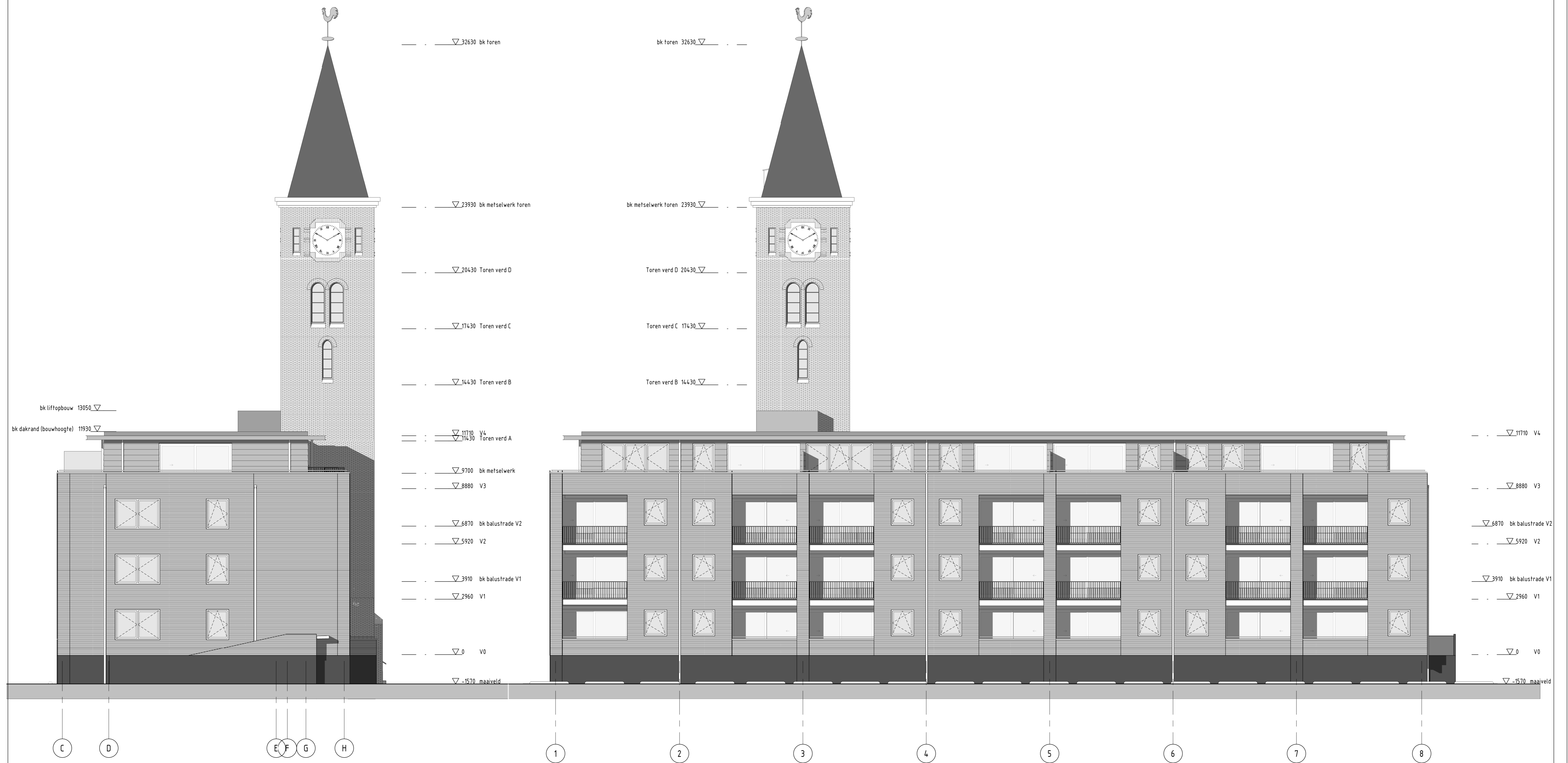
Zuidgevel schaal 1:100
