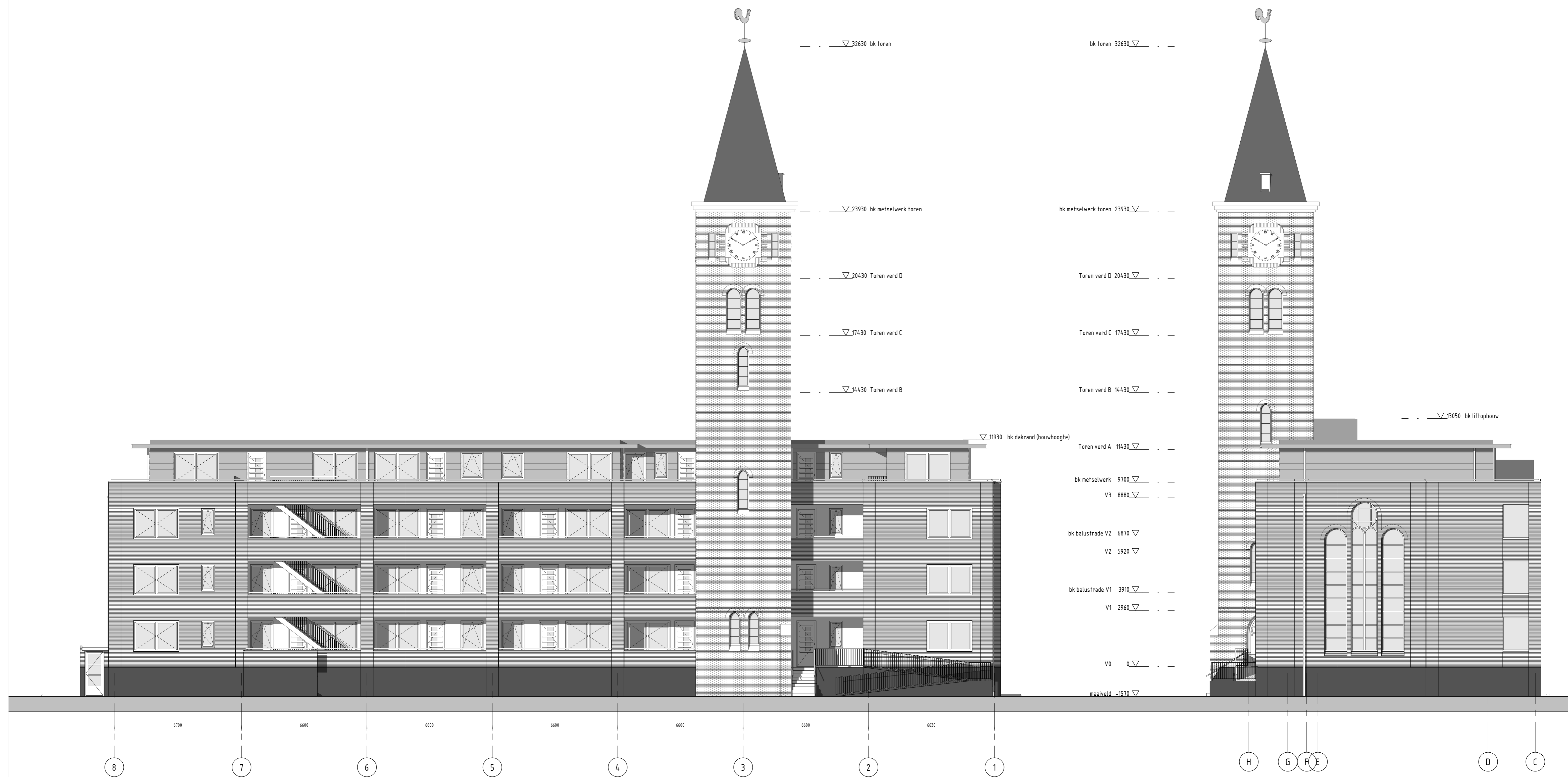
Oostgevel schaal 1:100
