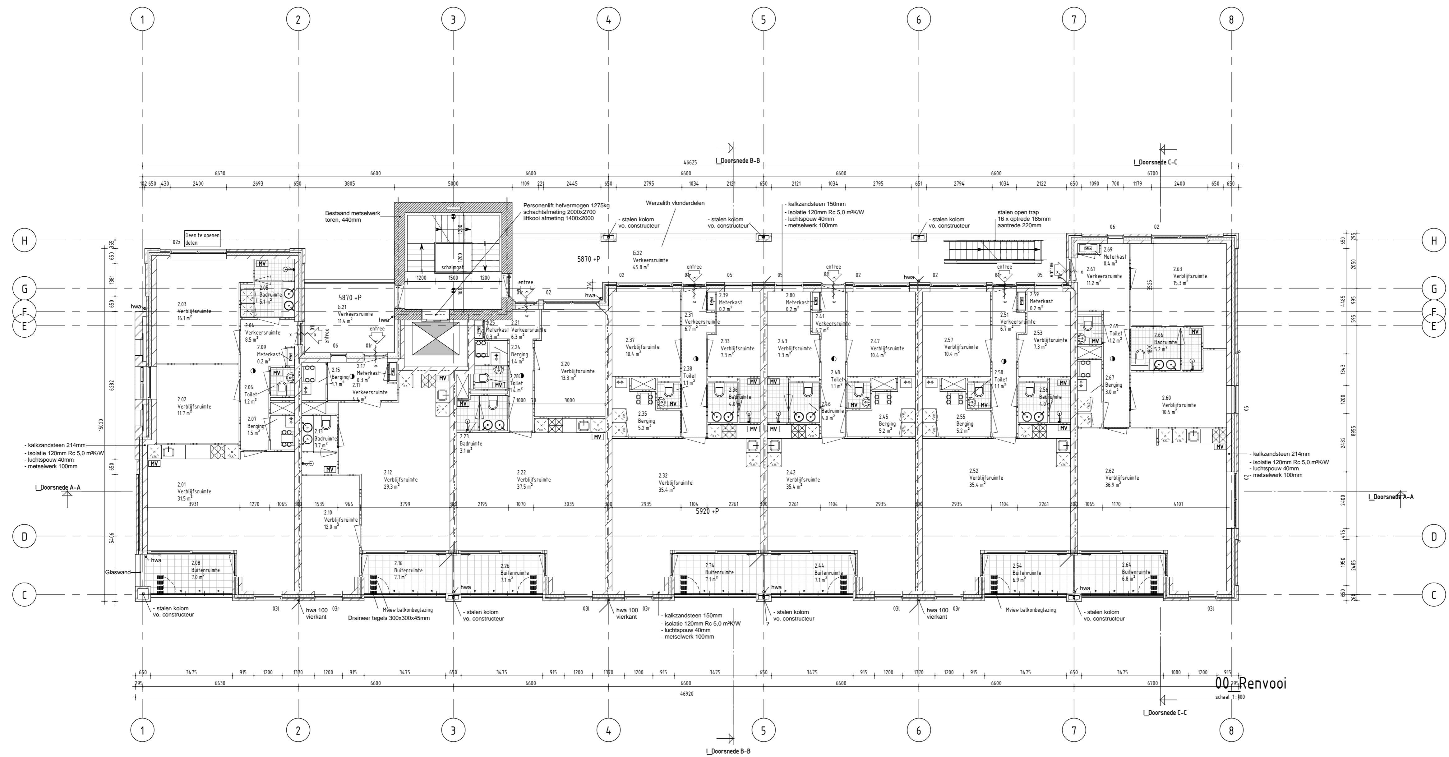
Plattegrond Tweede Verdieping schaal 1:100
