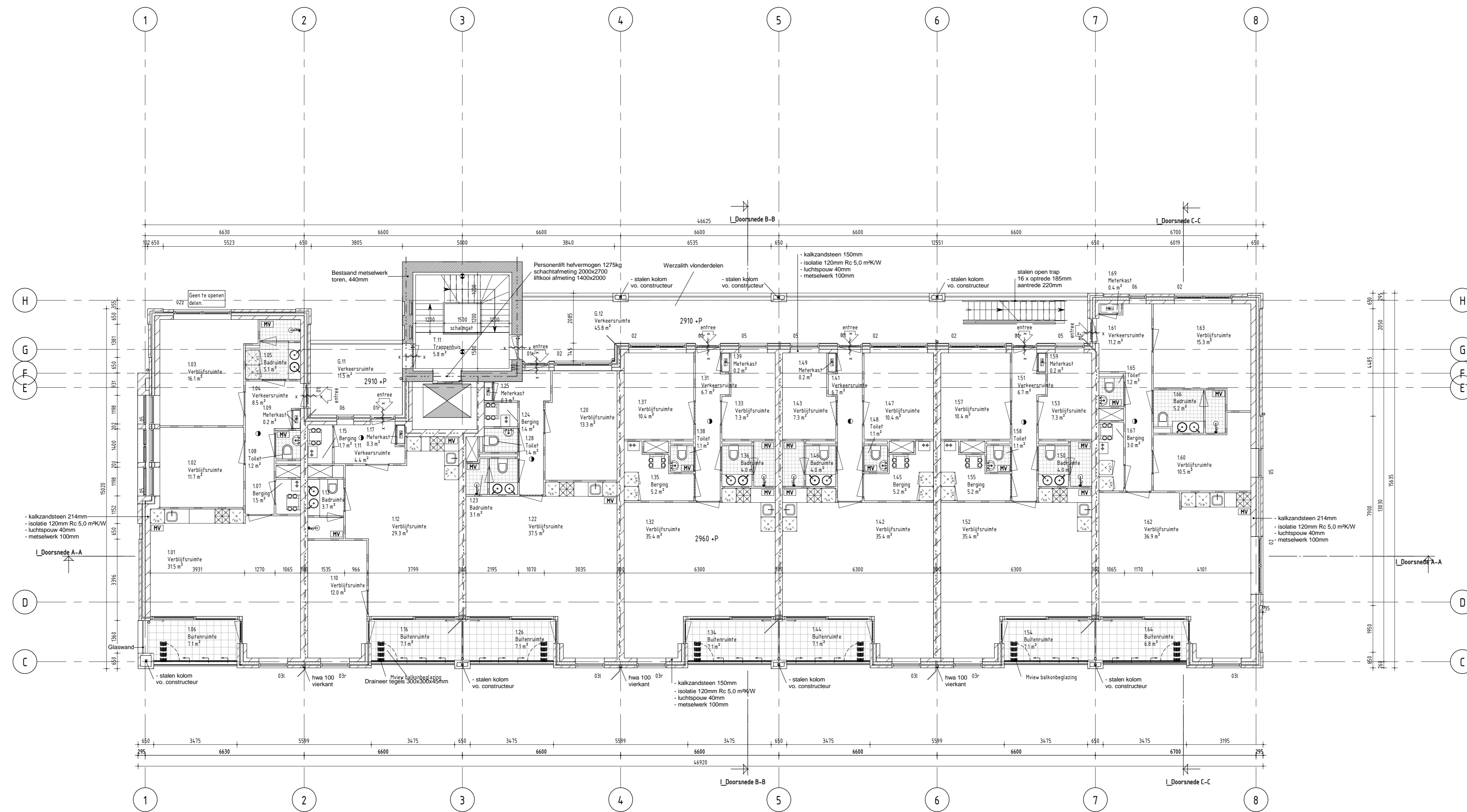
Plattegrond Eerste Verdieping schaal 1:100
