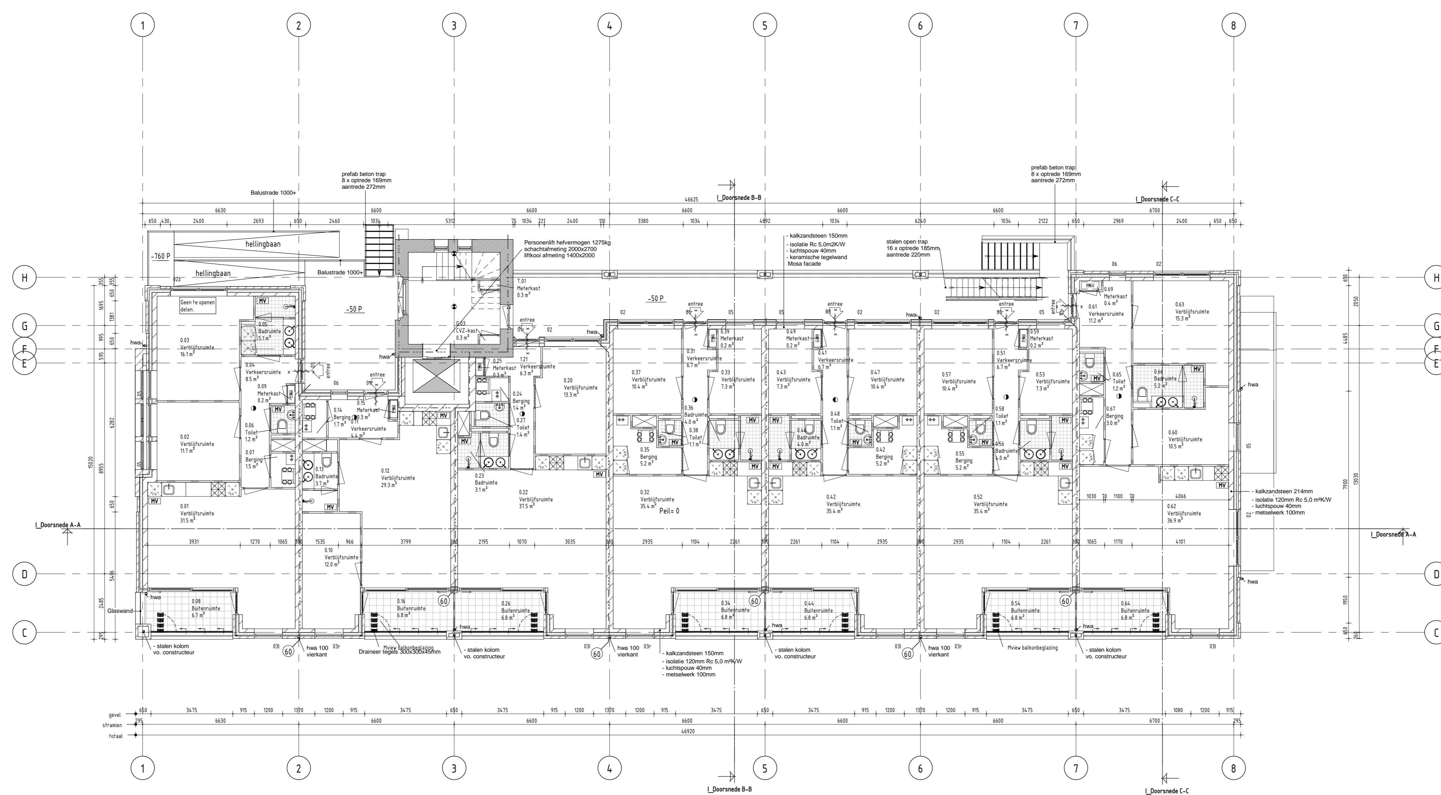
Plattengrond Begane Grond schaal 1:100
