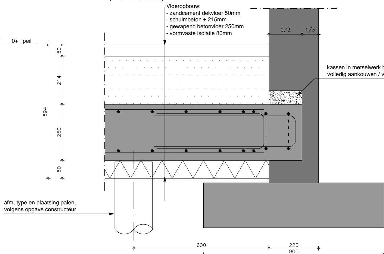
standaard vloerrand tpv inkassing (nieuwe situatie) inlaagpolder 5
