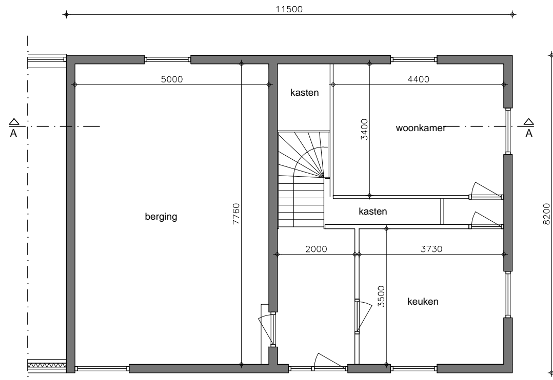
begane grond (Bestaande situatie)
