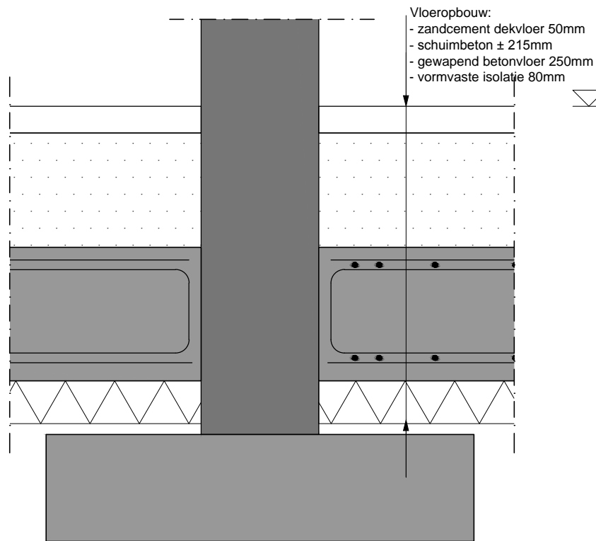
standaard vloerrand binnenmuur (nieuwe situatie)
