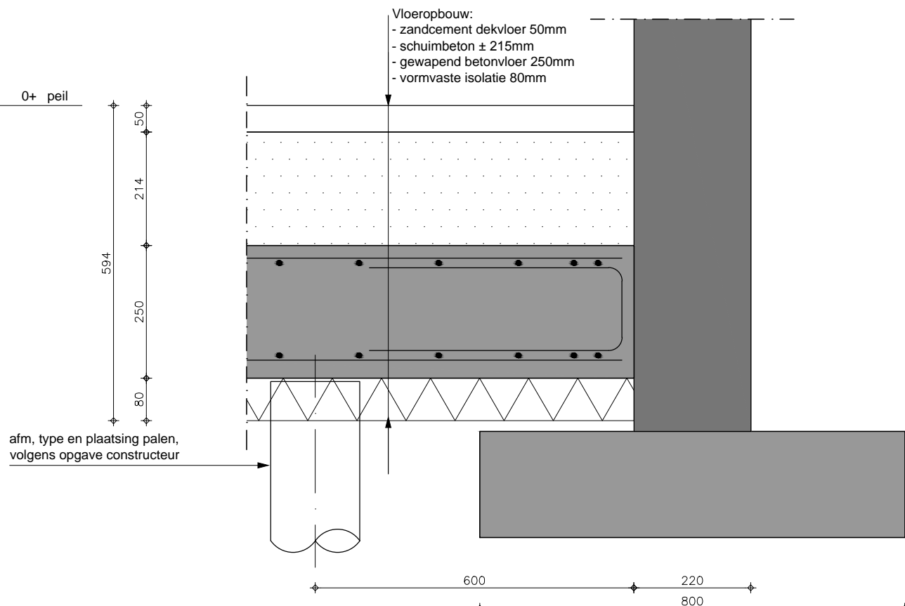
standaard vloerrand (nieuwe situatie)
