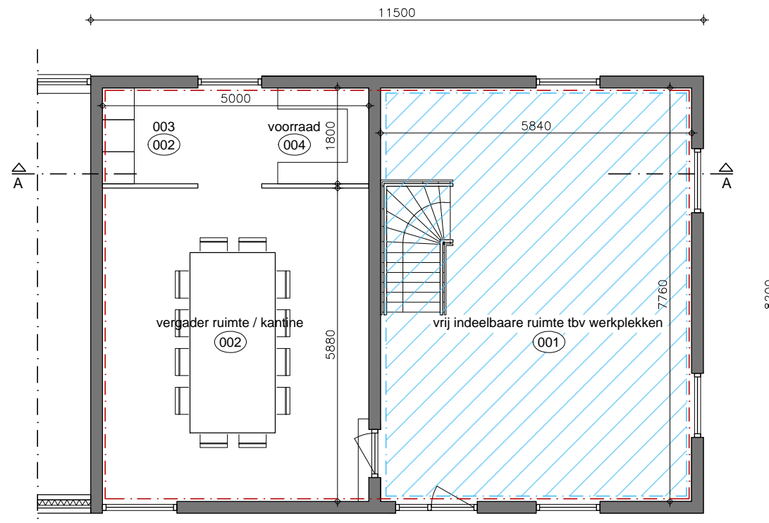
begane grond (nieuwe situatie)
