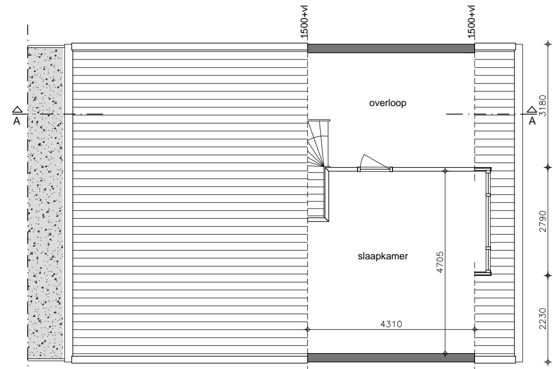
eerste verdieping (Bestaande situatie)
