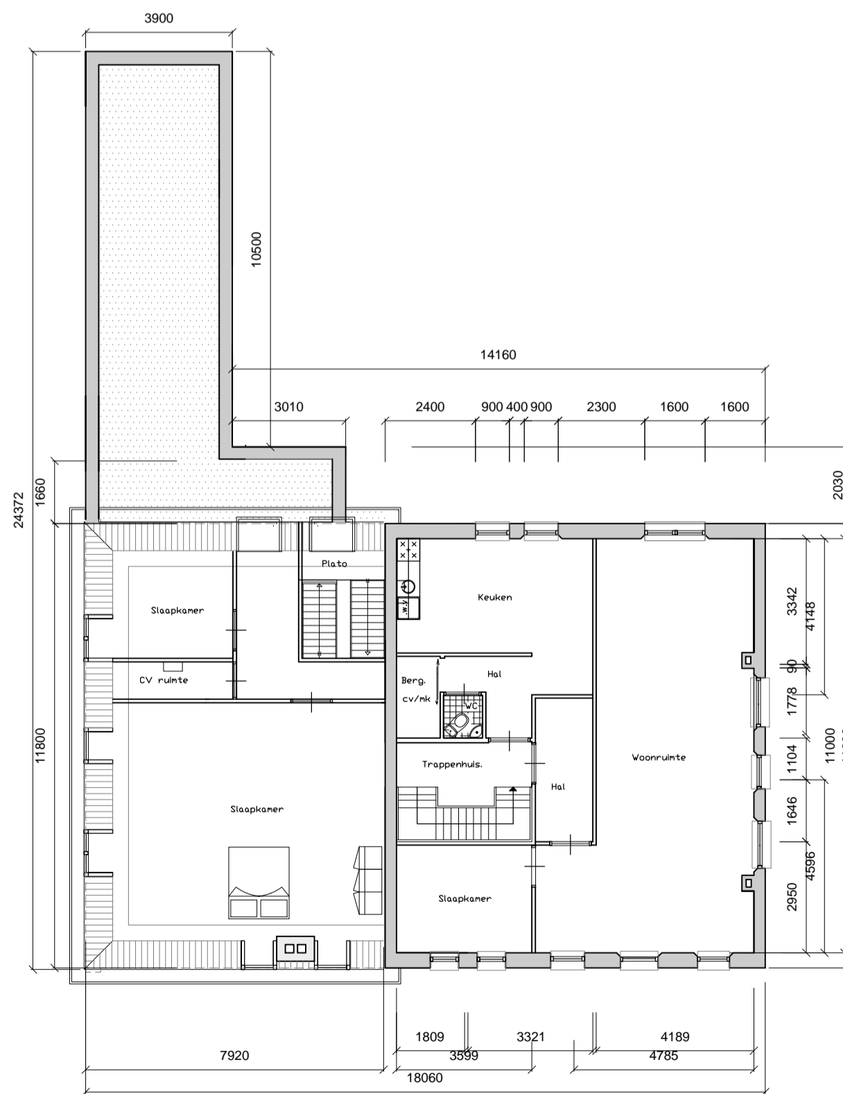
1e verdieping
