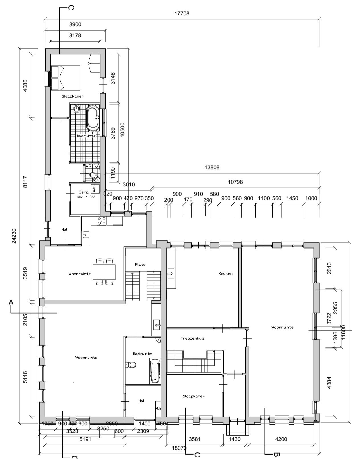
begane grond
