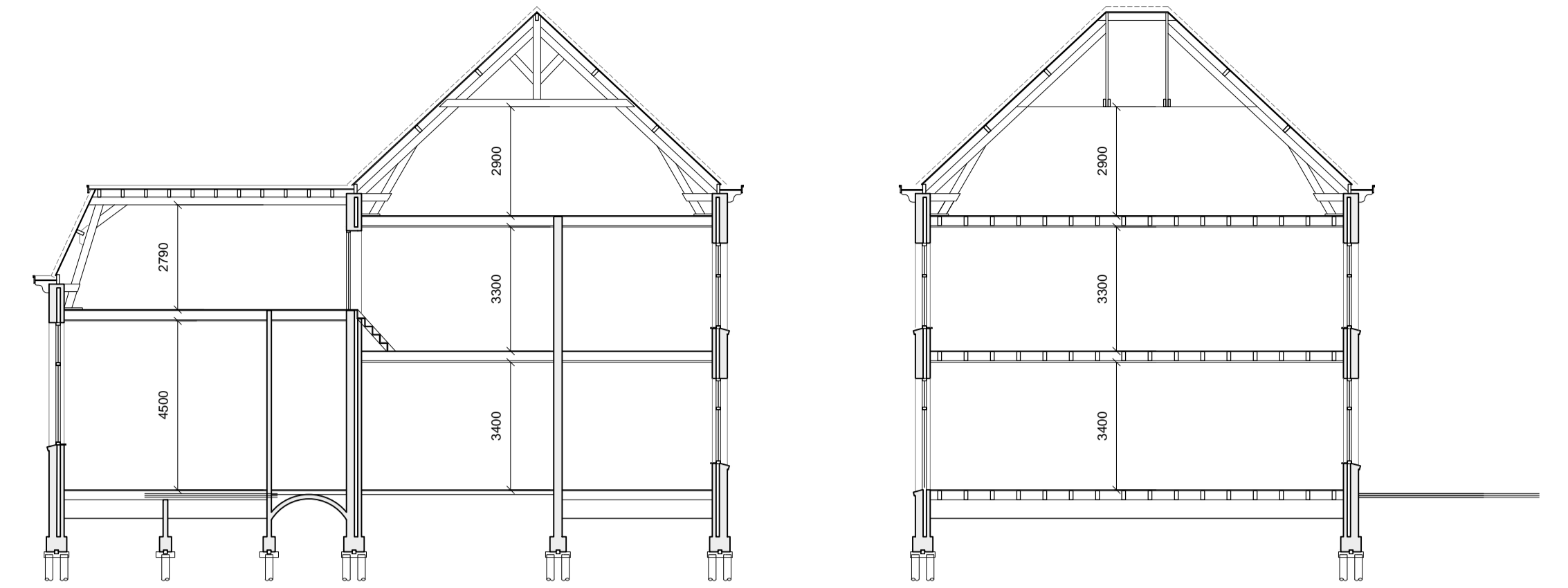
hoogtedoorsnede A - A
