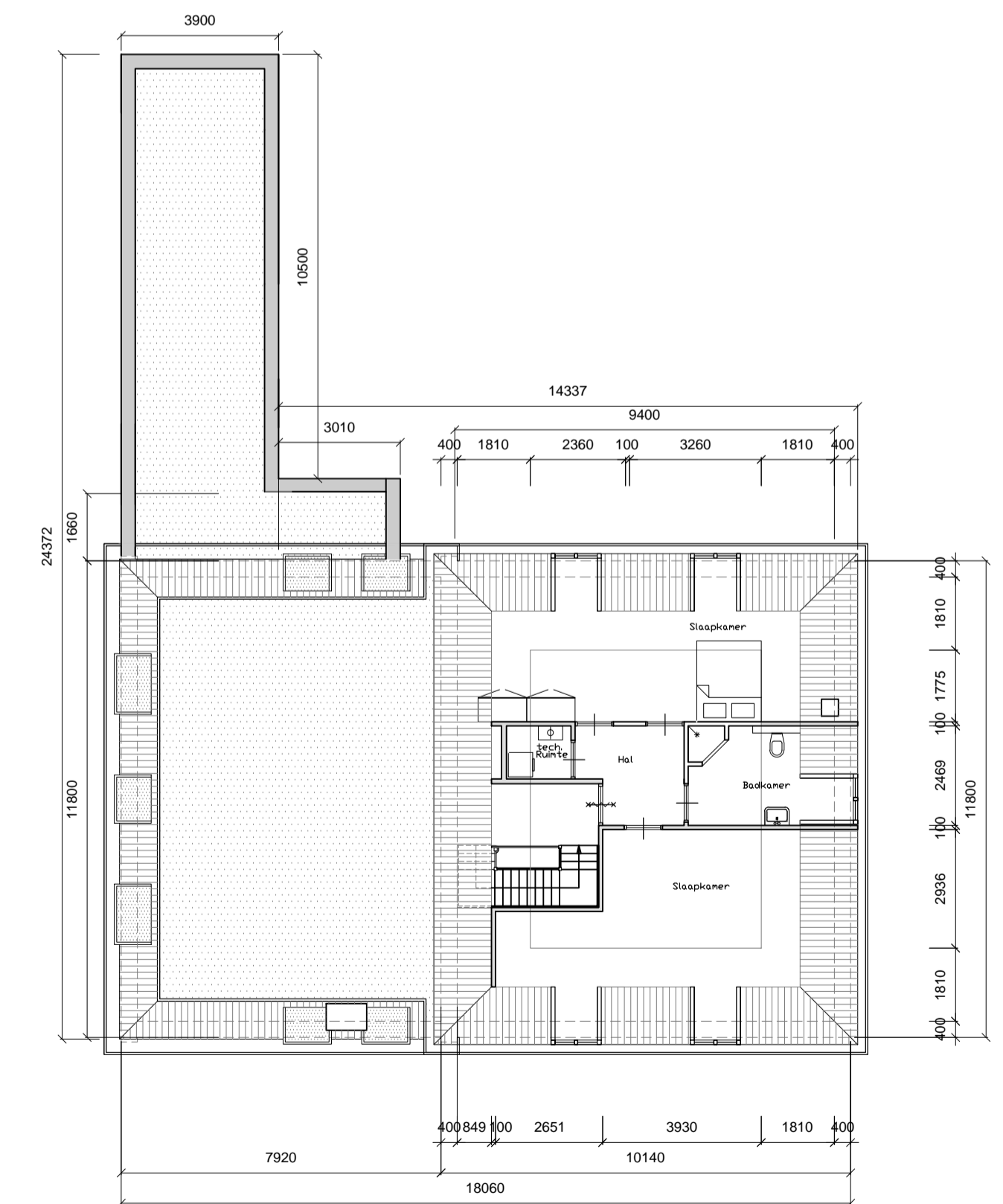
2e verdieping
